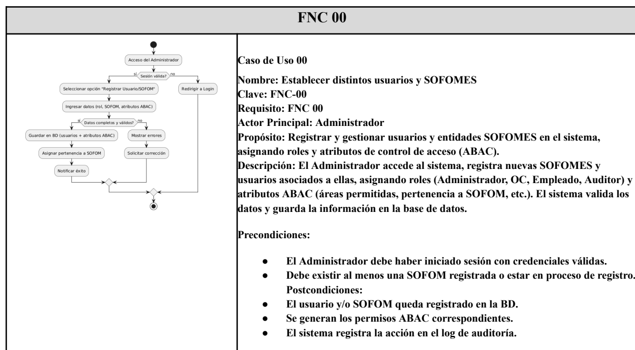
Figura 1. Detalles del Caso de Uso 00 y Diagrama de Actividades.
