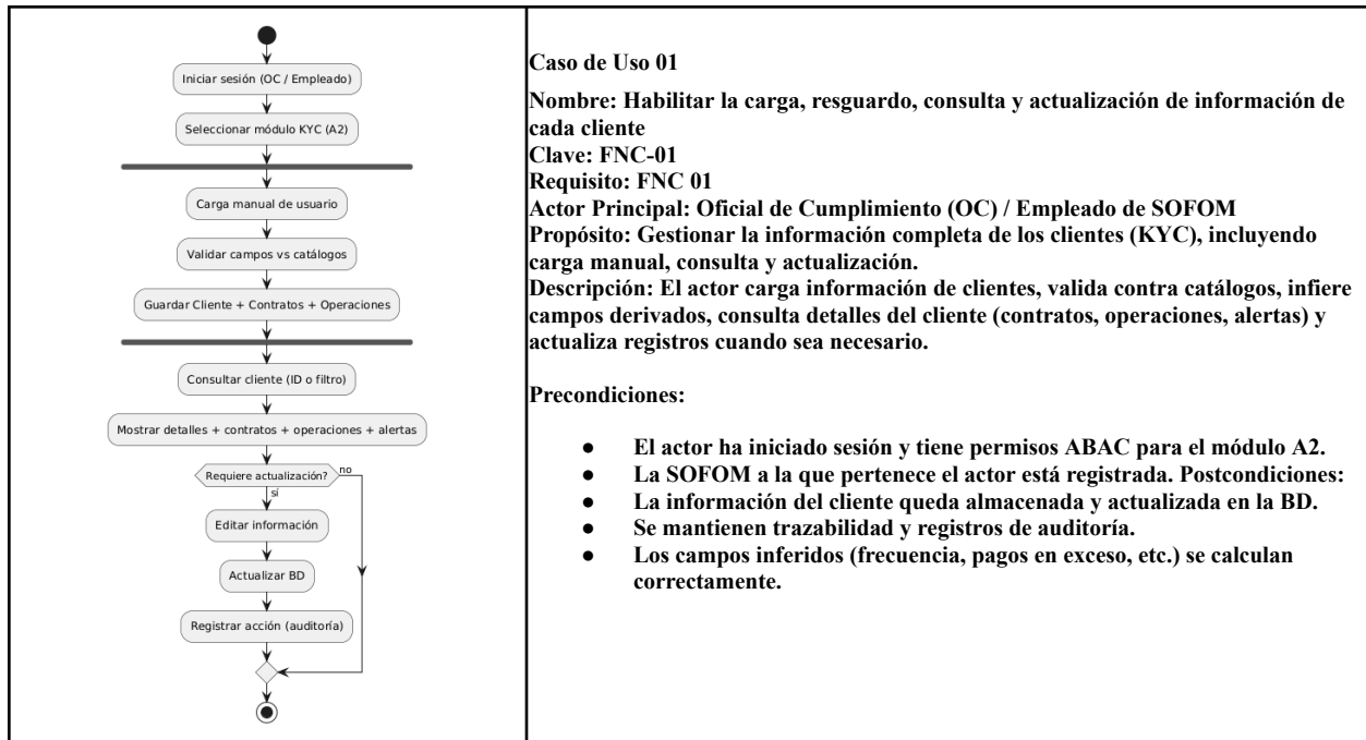
Figura 2. Detalles del Caso de Uso 01 y Diagrama de Actividades
