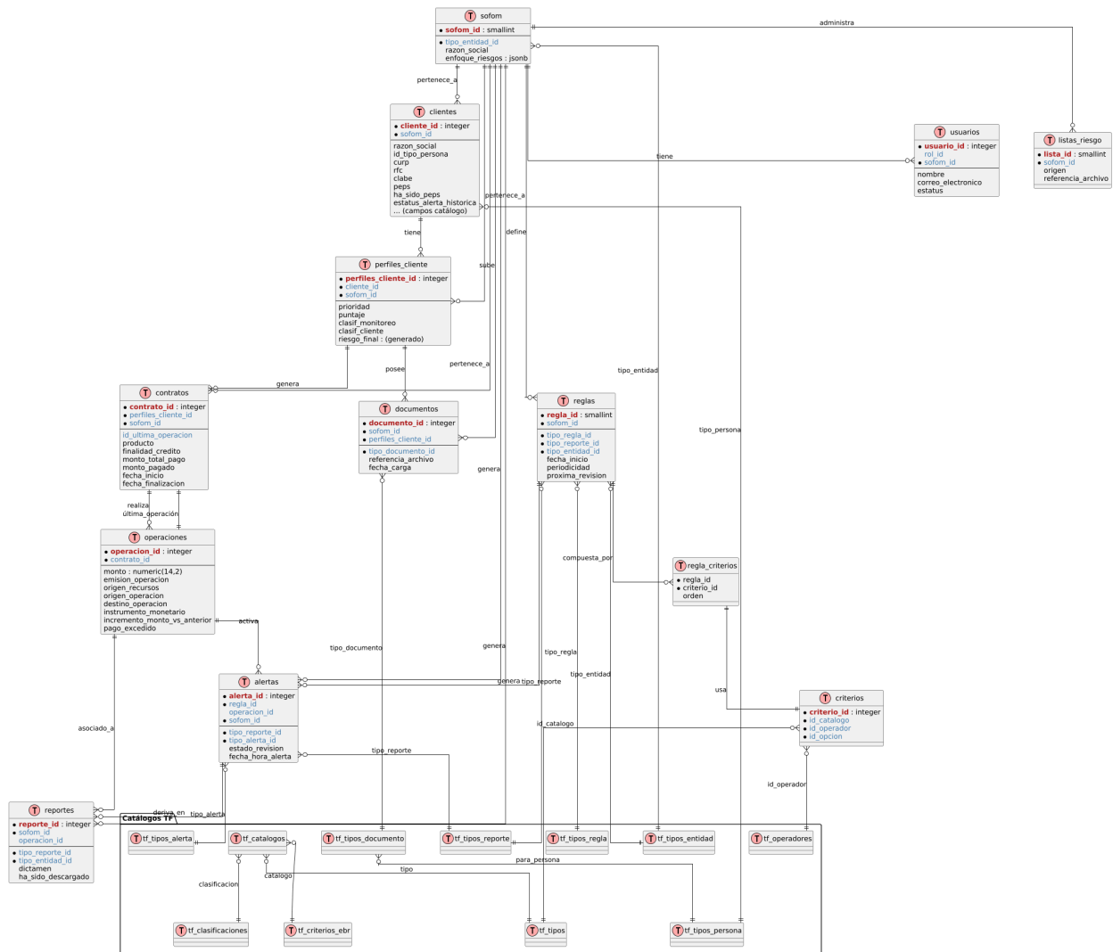
Figura 7 - Modelo Entidad-Relación para Sistema Automático SVA Law.
