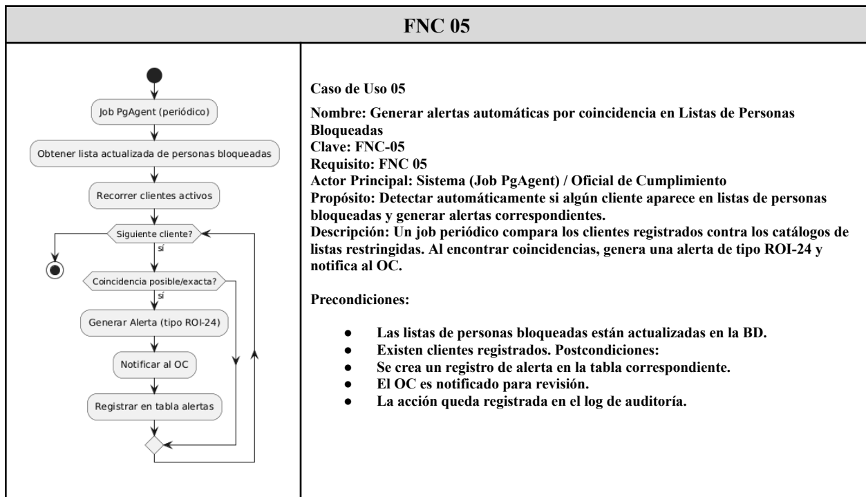
Figura 3. Detalles del Caso de Uso 05 y Diagrama de Actividades
